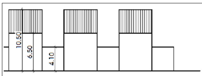
Systemskizze: Höhenentwicklung der Kettenhausbebauung im Baugebiet WA1.2 des rechtskräftigen Bebauungsplans „Hintere Heide II – 8. Änderung“
