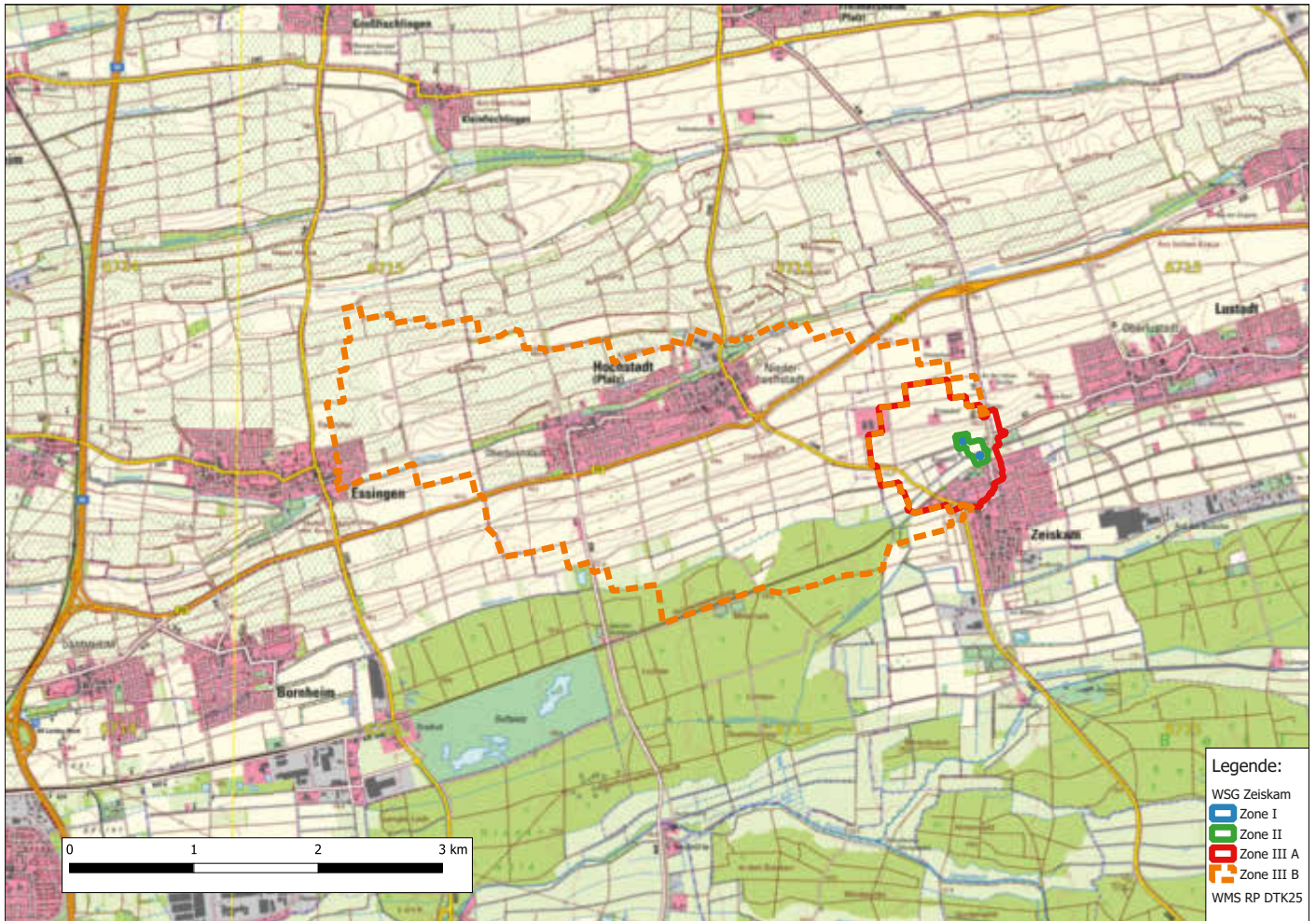
WSG Zeiskam Übersicht - Lageplan (ohne Maßstab)
