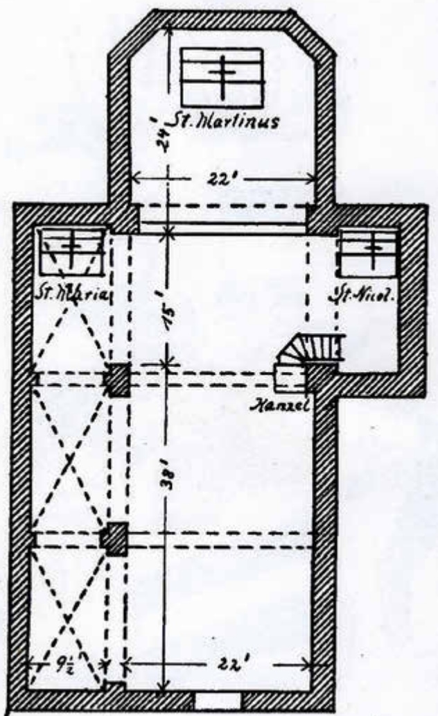
Plan der alten Kirche nach Joh. Weber
