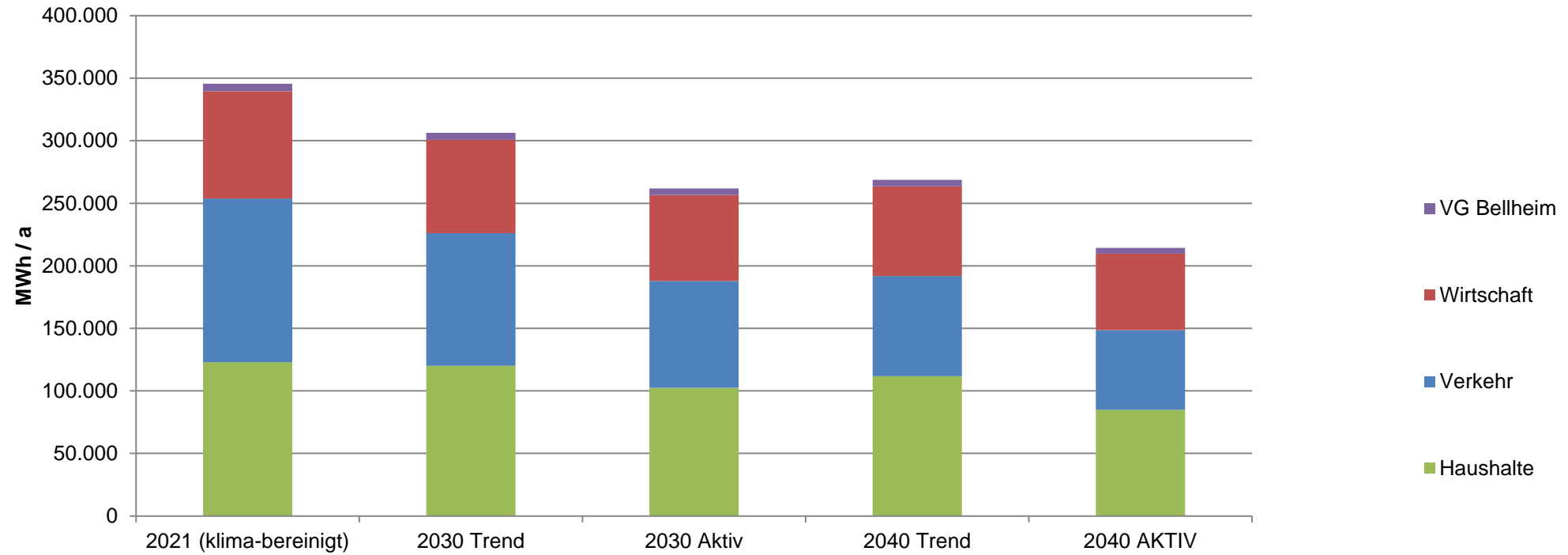
Entwicklung des Energieverbrauchs nach Verbrauchssektoren
